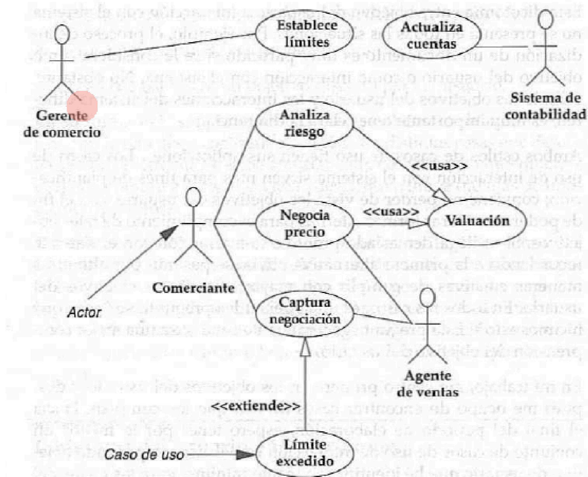
Figura 3-1: Diagrama de casos de uso
